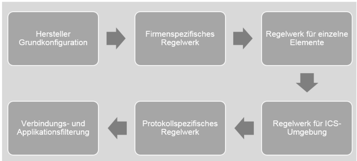
Abbildung 17 Vorgehen bei der Implementierung einer Firewall
