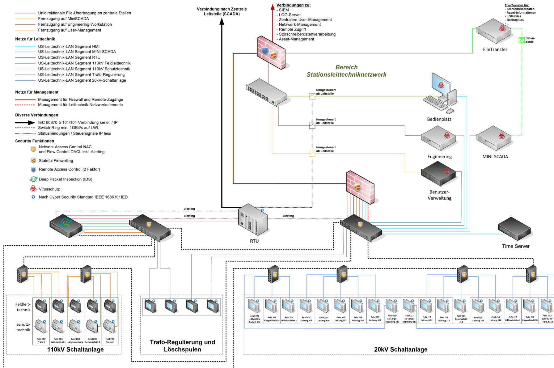
Abbildung 21 Beispiel für System-Aufbau einer versorgungskritischen Anlage
