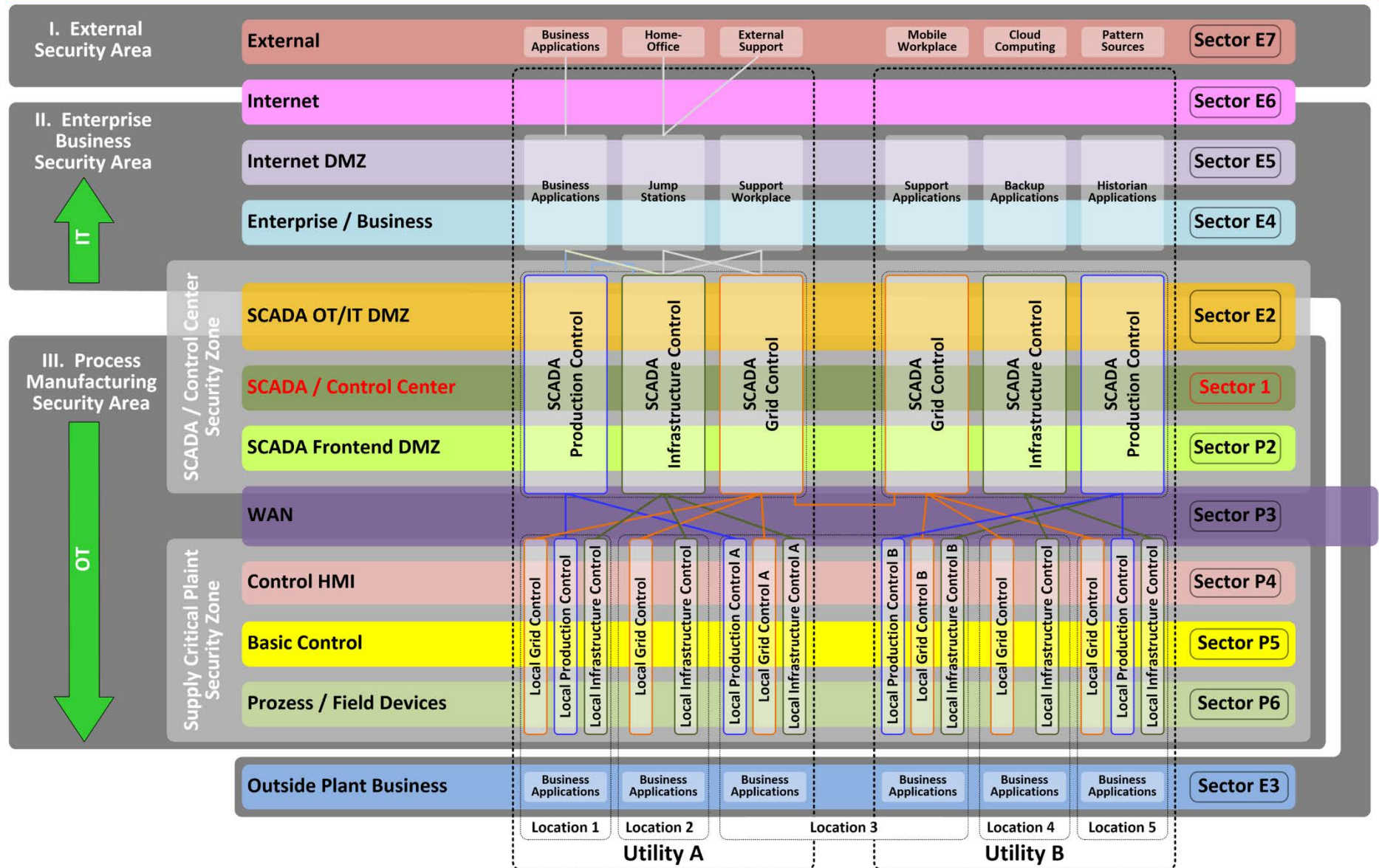
Abbildung 12 Systemlandschaft im ICS Umfeld
