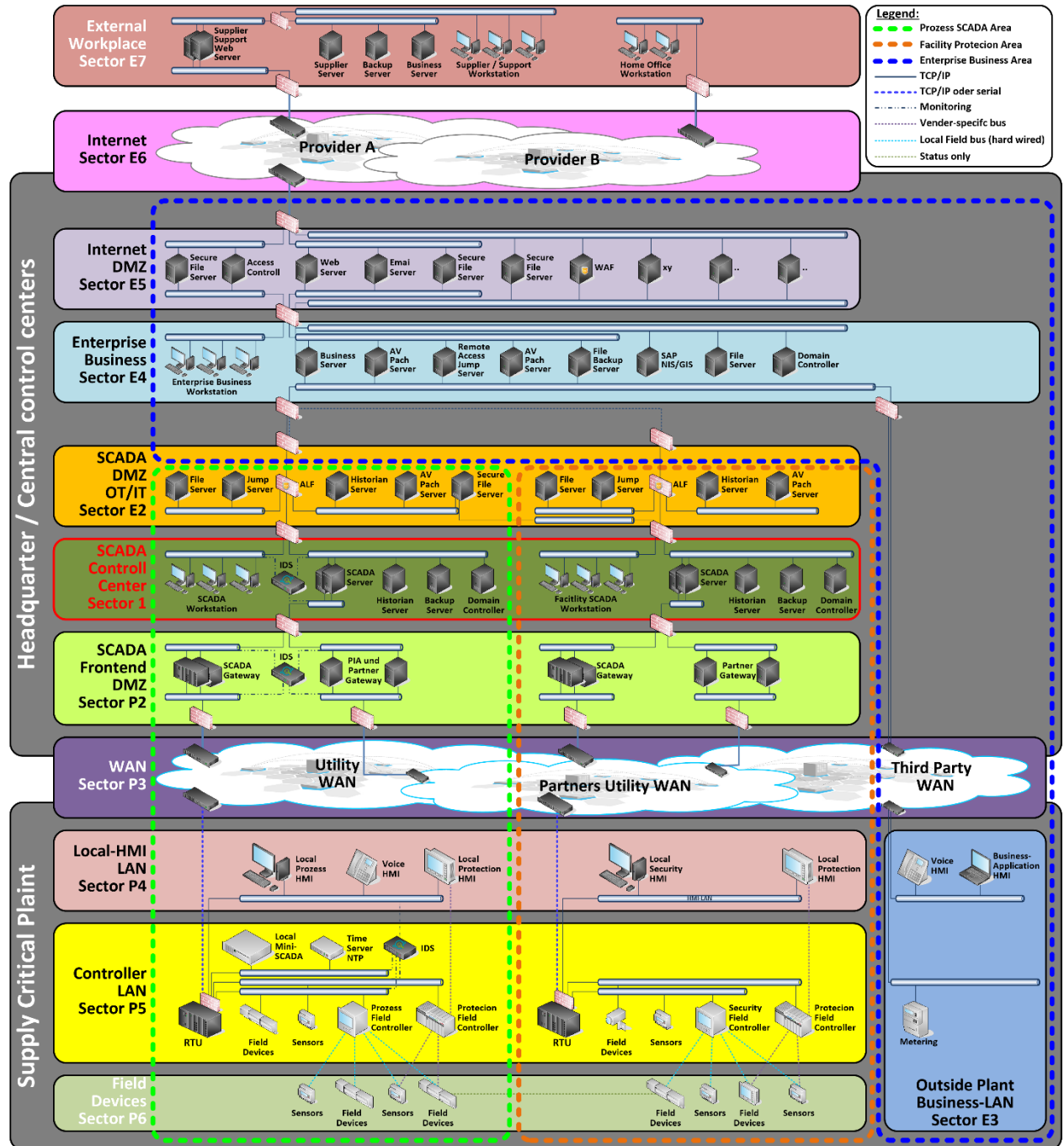
Abbildung 16 Empfohlene sichere Netzwerkarchitektur
