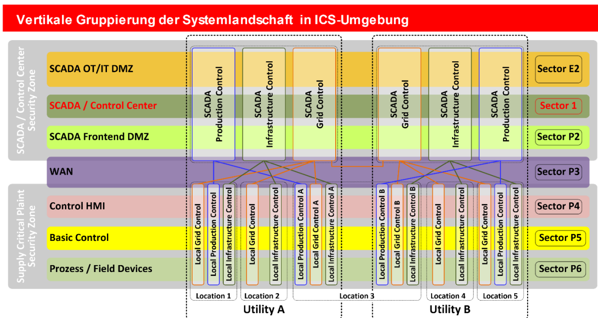
Abbildung 13 Vertikale Gruppierung der Systemlandschaft in ICS-Umgebung
