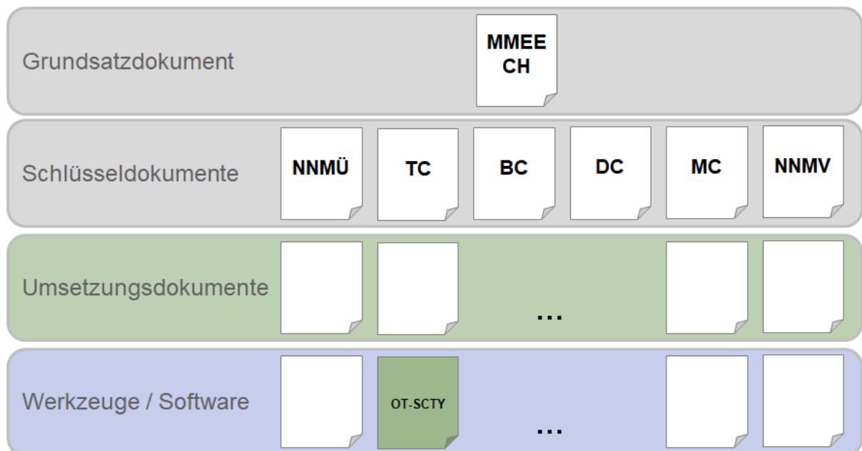
Abbildung 1 Dokumentstruktur
