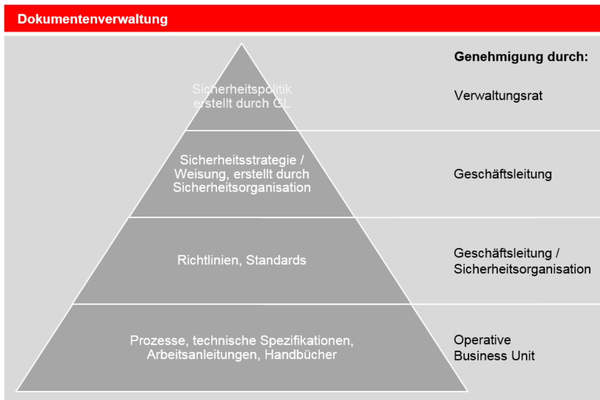
Abbildung 6 Dokumentenhierarchie
