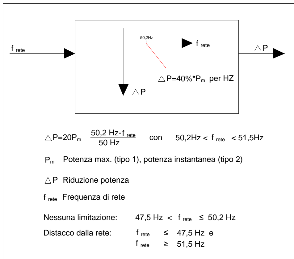
Figura 19: Riduzione della potenza in caso di sovrافrequenza nella media tensione (TC-CH 2013)
