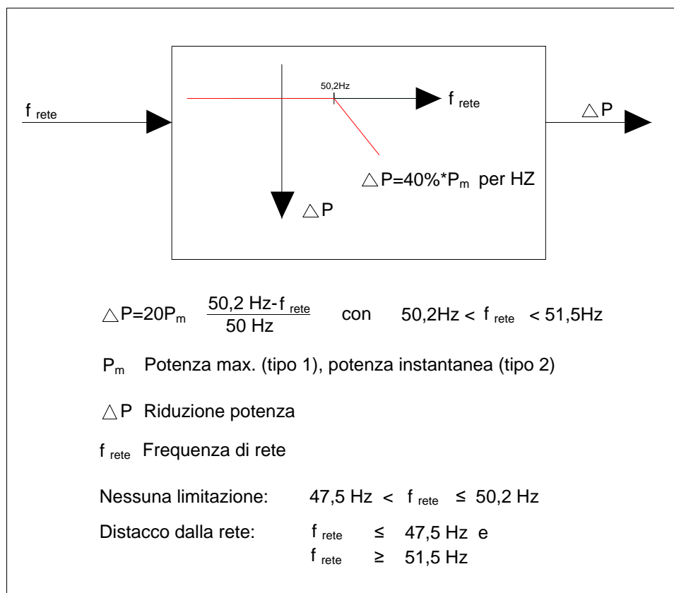
Figura 27 Riduzione della potenza in caso di sovralfrequenza nella bassa tensione (TC-CH 2013)
