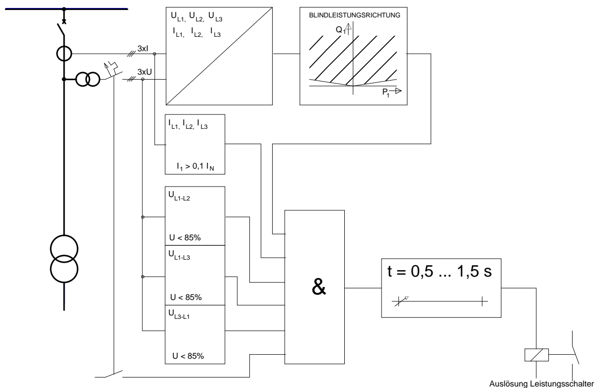
Abbildung 6: Beispiel Q-U-Schutz
