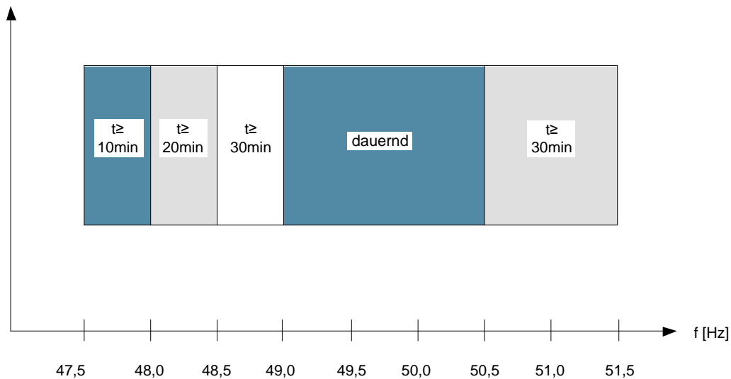
Abbildung 29: Frequenzbänder in der Niederspannung (Basis TC-CH 2013)
