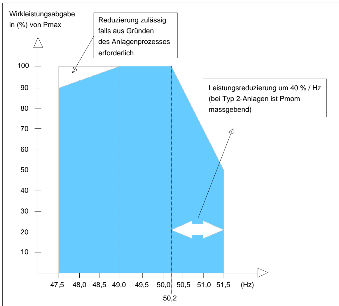
Abbildung 8: Übersicht von frequenzabhängigen Leistungsreduktionen
