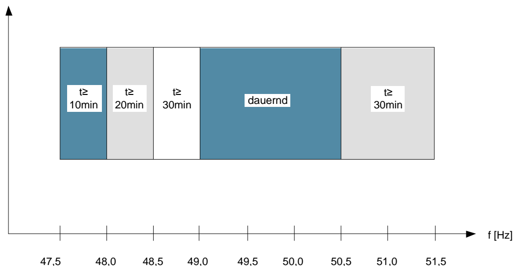
Abbildung 21: Frequenzbänder in der Mittelspannung (Basis TC-CH 2013)
