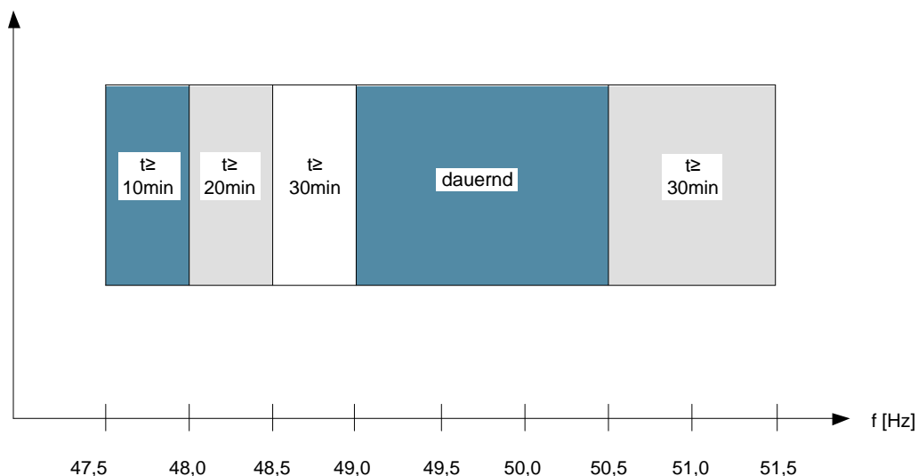
Abbildung 9: Frequenzbänder in der Hochspannung (Basis TC-CH 2013)
