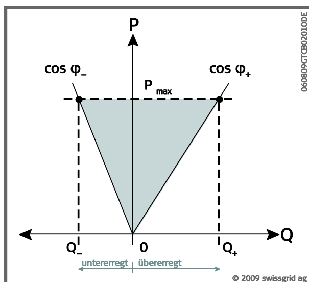
Abbildung 2: Anforderung am Anschlusspunkt an die Erzeugungseinheit für die Teilnahme an der Spannungsregelung (Erzeugerzählpeilsystem)
